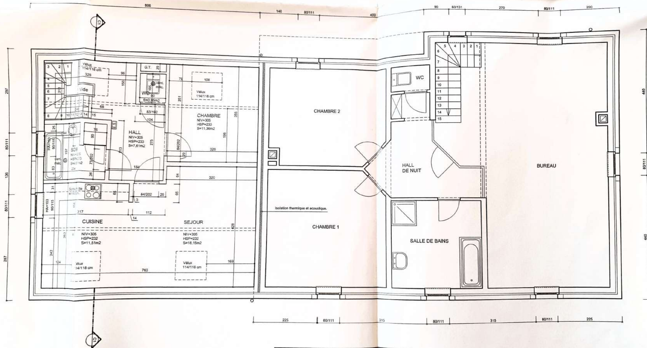
PLAN PREMIER ETAGE
